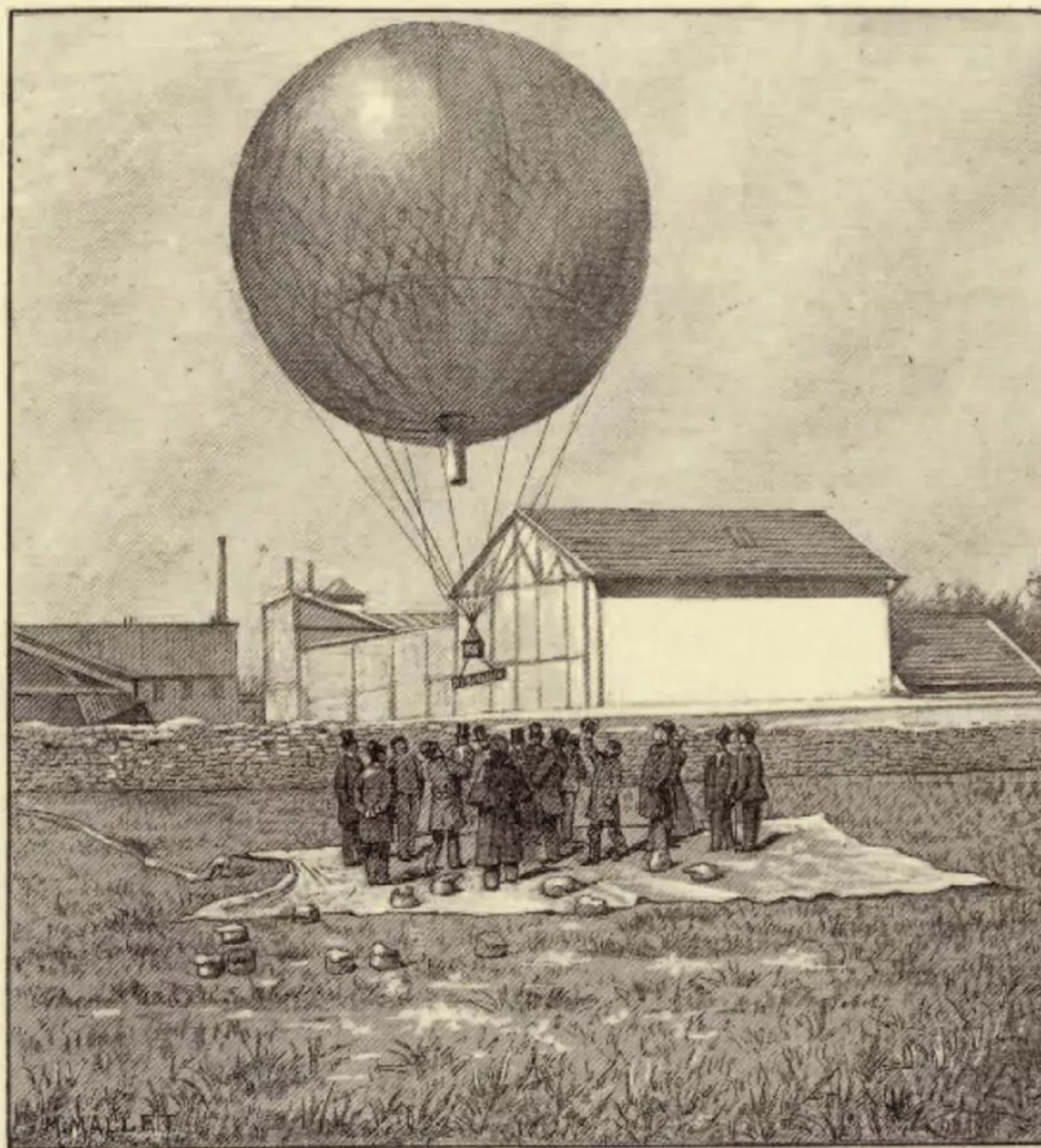
Le ballon-sonde Aérofile I décolle du parc de Vaugirard, à Paris, le 21 mars 1893. Il atteindra l'altitude de 16 000 mètres et enregistrera la température la plus basse jamais constatée : - 57 °C.
