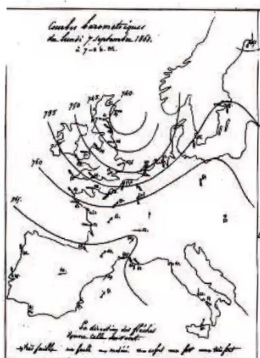
La première carte barométrique française, établie en 1863 par Le Verrier et Marié-Davy et publiée dans le Bulletin de l'Observatoire impérial .
