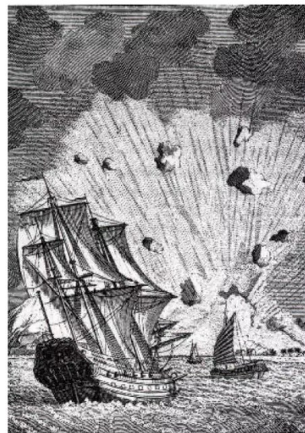
Le volcan Tambora s'embrase, provoquant en Europe une « année sans été ».
