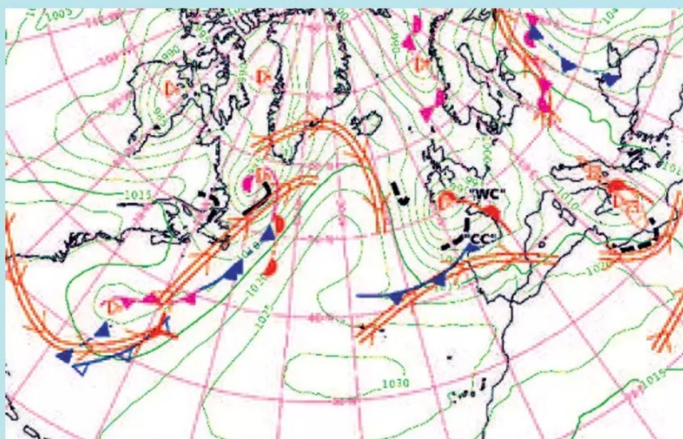
CARTE SYNTHÉTIQUE Les traits verts figurent les courbes isobares, reliant les points de pression égale; les D rouges, les dépressions; les fronts sont repérés en rouge (chaud) et bleu (froid). C est le nom de l'onde pluvieuse, chaude (WC) ou froide (CC); les traits orange indiquent le courant-jet d'altitude.
