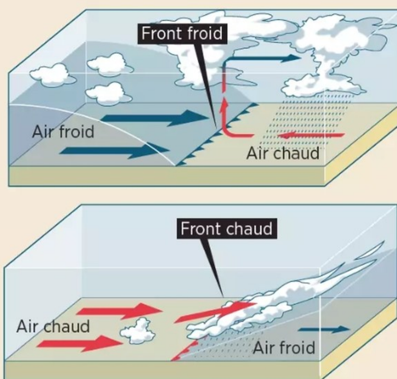
Fronts froids et chauds rythment les températures et les précipitations.
