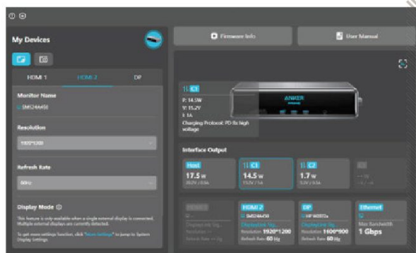
◀ Depuis l'interface PC, il est possible de connaître le protocole de charge de chaque terminal connecté en USB-C.
