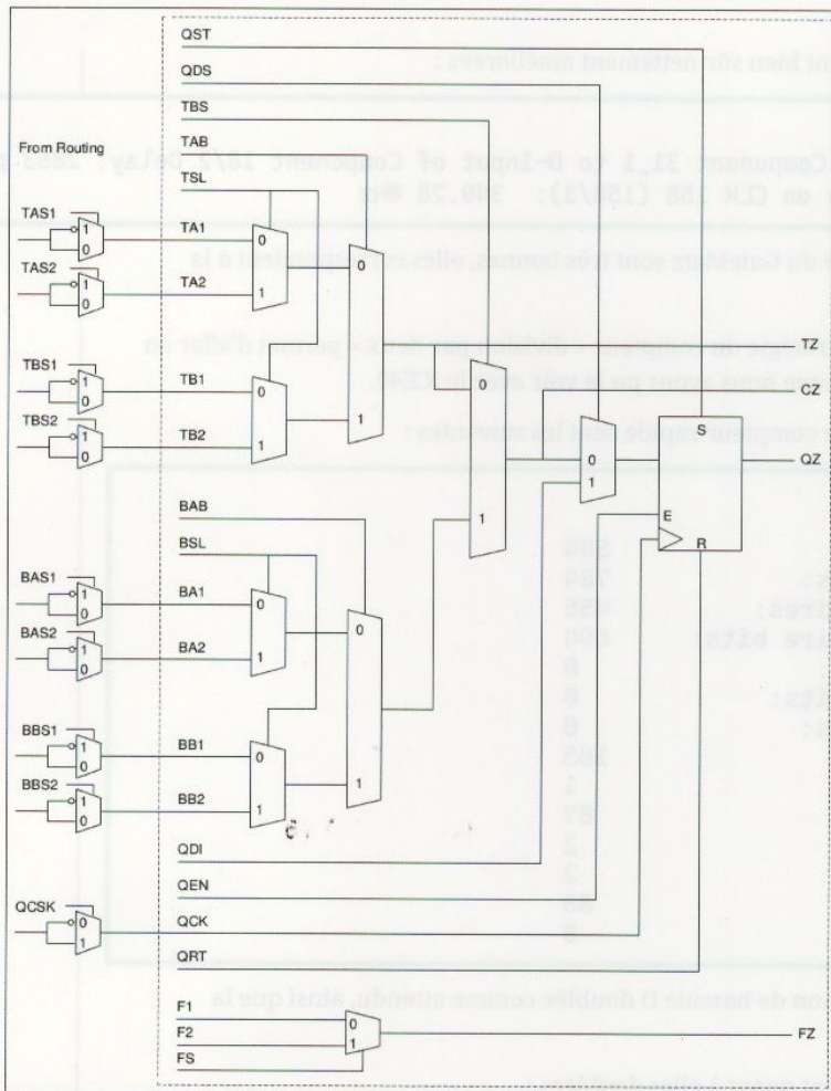
Fig. 10 : La cellule logique de base du eFPGA de l'EOS S3 a la spécificité de ne pas utiliser de LUT mais des multiplexeurs.
