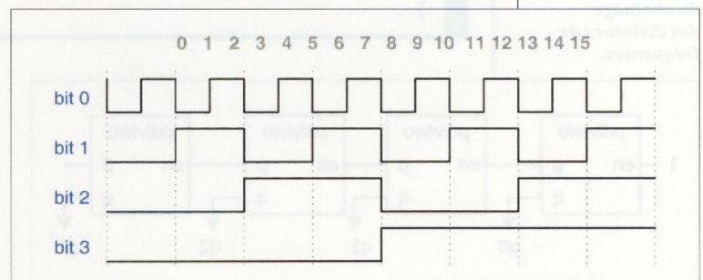
Fig. 1 : Un compteur naturel n'est en fin de compte qu'un ensemble d'horloges carrées dont la fréquence est divisée par 2 à chaque bit.
