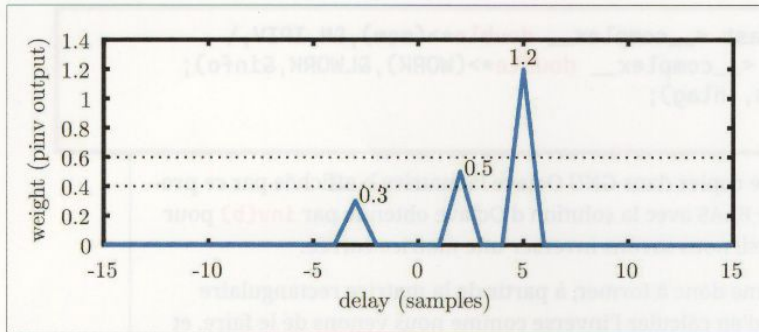
Figure 6 : Module du produit de la pseudo-inverse de la matrice contenant les copies retardées de l'interférent connu avec le signal bruité observé, contenant ce code pour des retards de -3 échantillons, +2 et +5. Comparer avec la Fig. 5 : cette fois, une estimation quantitative des retards et pondérations est fournie par la pseudo-inverse dont les résultats sont en accord avec les valeurs utilisées lors de la synthèse du signal.
