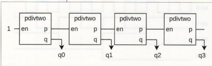
Fig. 3 : Schéma du chaînage des diviseurs de fréquences.
