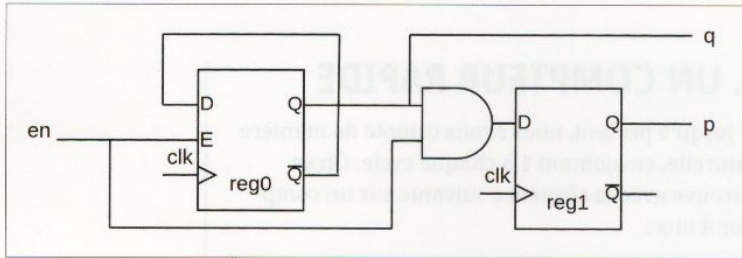
Fig. 2 : Schéma du diviseur de fréquences par deux, il n'y a qu'une porte entre deux bascules D. Même si l'on agrandit le compteur, le chemin critique reste constant.
