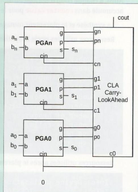
Fig. 15 : Plutôt que de chaîner chaque sortie de retenue sur l'entrée du bloc suivant, on délègue le calcul au bloc CLA qui anticipera le calcul de toutes les retenues.
