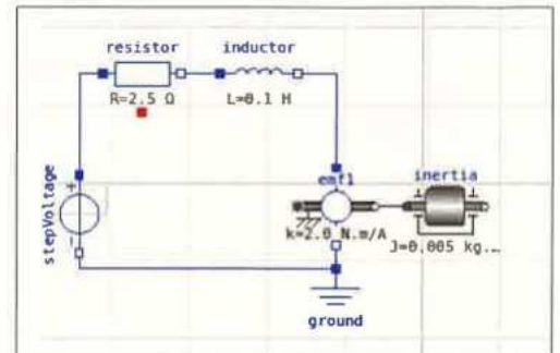
Figure 8 : Modèle du moteur électrique.
