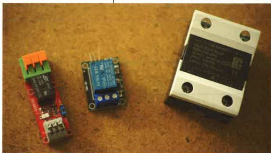
Fig. 2 : Des relais compatibles avec la tension de sortie de nos modules (3 V, avec éventuellement une borne en +5 V non programmable). De gauche à droite : un relais 20 A/14 VDC, un relais 10 A/230 VAC, un relais SSR 120 A/230 VAC. Attention avec ce dernier : il nécessite un radiateur pour fonctionner.
