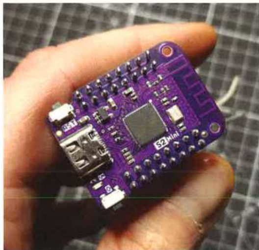
Le module ou carte Wemos S2 Mini est relativement minimaliste et repose entièrement sur les fonctions fournies par le SoC ESP32-S2FN4R2 intégrant un contrôleur USB (USB CDC ACM), la flash et la PSRAM. En dehors d'un quartz, d'un régulateur de tension et de quelques composants passifs, cet ESP32 n'a besoin d'aucun autre élément pour fonctionner.
