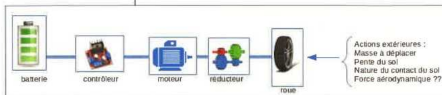
Figure 7 : Chaîne de traction.
