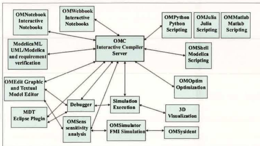
Figure 1 : Architecture de l'environnement OpenModelica [9].
