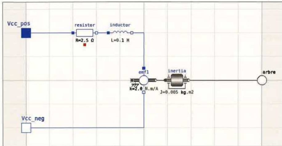
Figure 11 : Modèle du Moteur DC.
