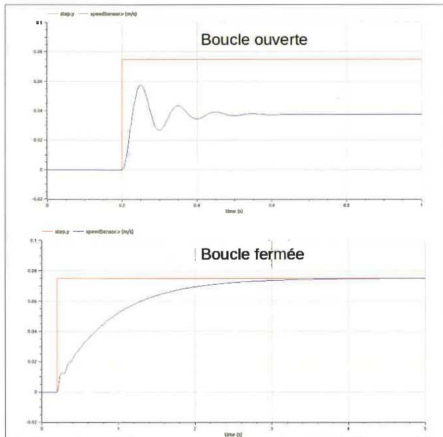
Figure 20 : Réponse indicielle en boucle ouverte et en boucle fermée.
