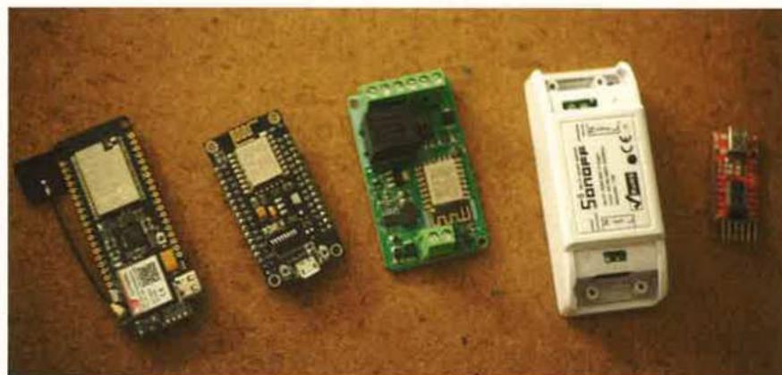
Fig. 1 : Plusieurs cartes possibles pour ce projet, de gauche à droite : le T-Call de LILYGO comporte un ESP32 avec son module SIM800L, le NodeMCU basé sur le microcontrôleur ESP8266, une carte ESP8266 avec un relais intégré, le module Sonoff (ESP8266 également, avec un relais), et un adaptateur FDTI USB vers port COM, nécessaire pour flasher les deux dernières cartes.
