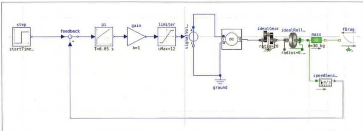
Figure 19 : Asservissement en vitesse du véhicule en boucle fermée.
