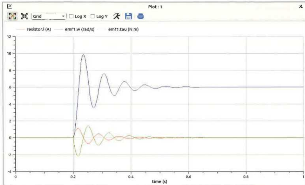
Figure 10 : Courant, couple et vitesse du moteur à vide.
