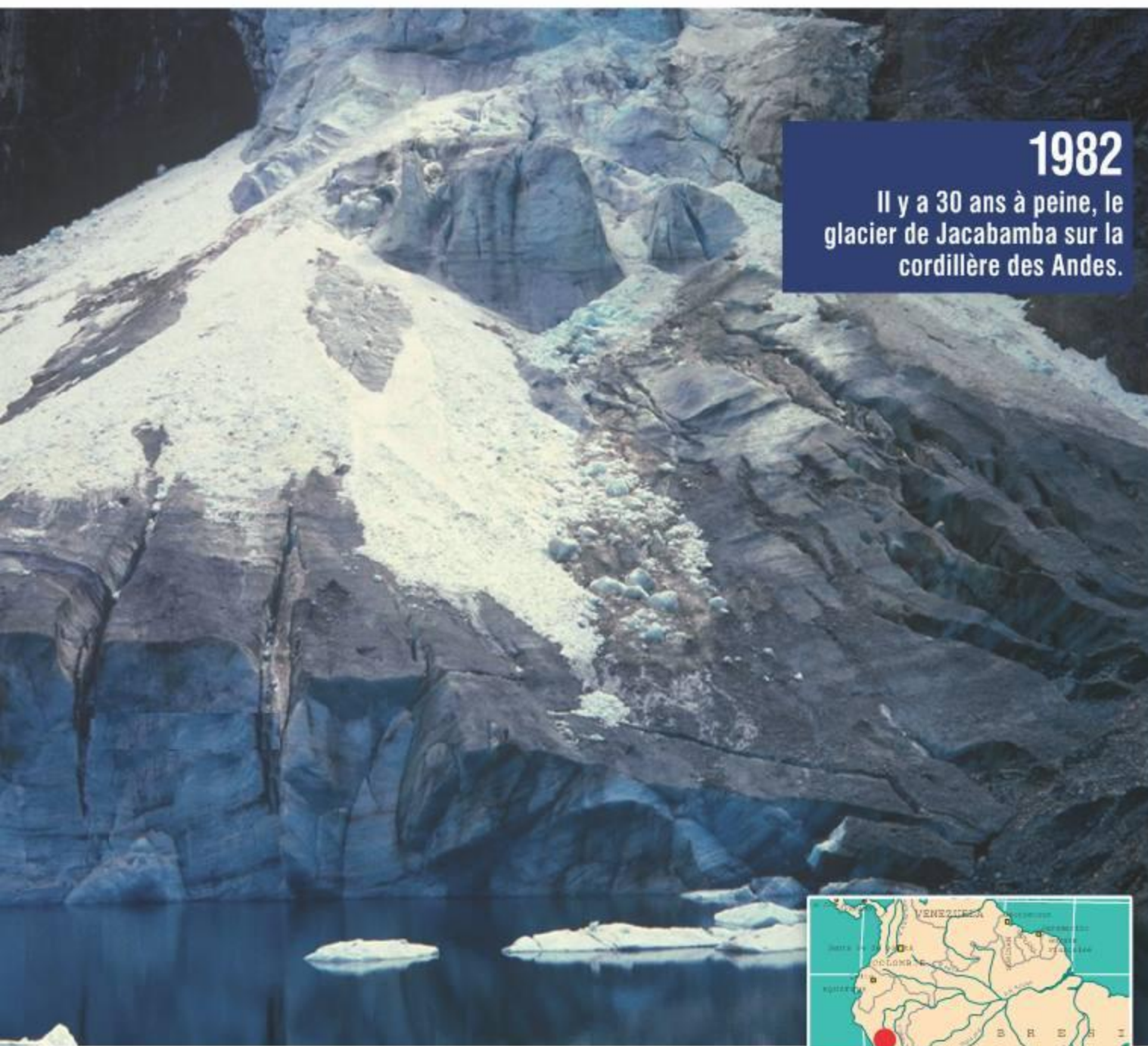
PÉROU Glacier de Jacabamba
