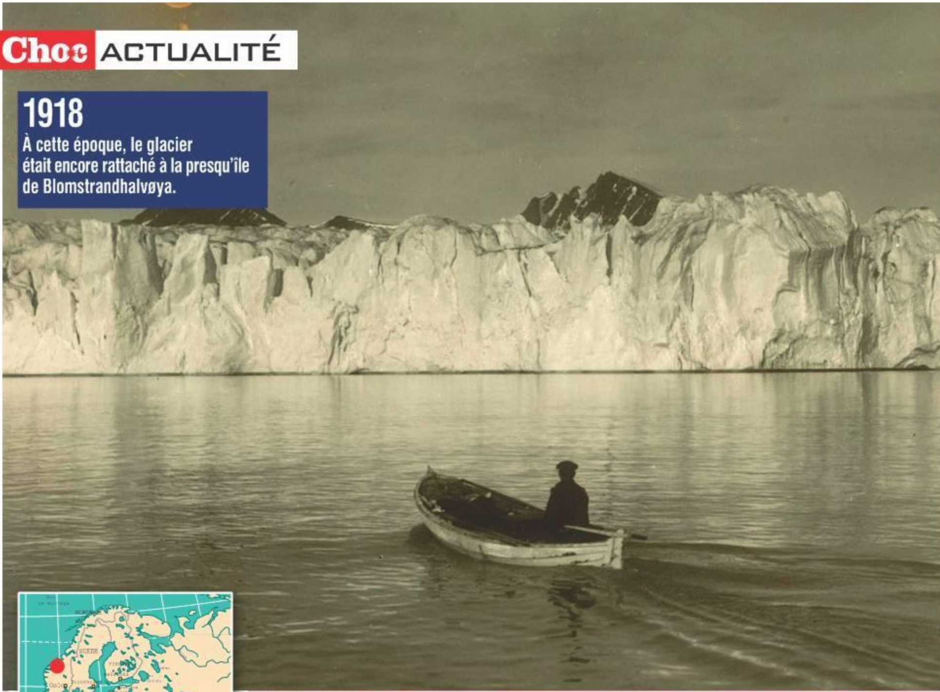
NORVÈGE Glacier Blomstrandbreen
